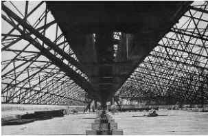
Hangar de Barajas y Talleres
